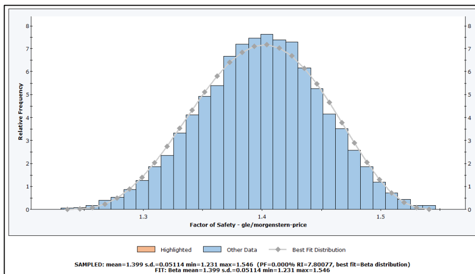
Figura 3.1. Histograma do Fator de Segurança – Cenário Atual
