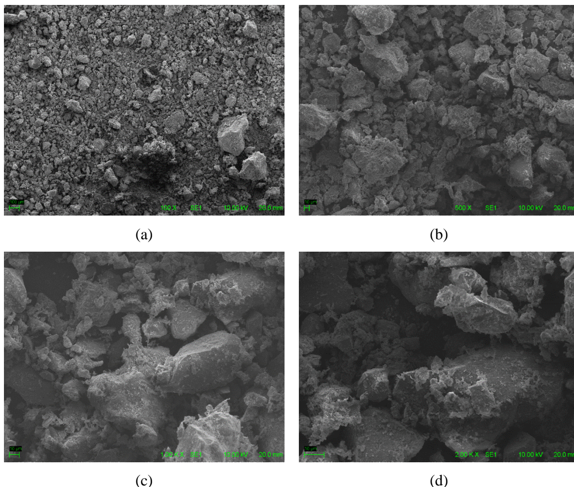
Figura 4 - Microscopia Eletrônica de Varredura do RMFB, nas magnificações: (a) 100x, (b) 500x, (c) 1000x e (d) 2000x.
