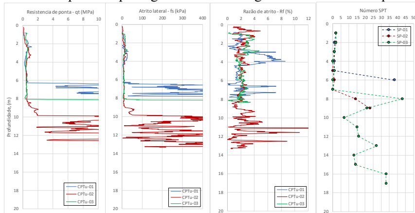
Figura 7. Resultados dos ensaios de campo ao longo do perfil do solo (SPT e CPTu) de Itajaí/SC.
