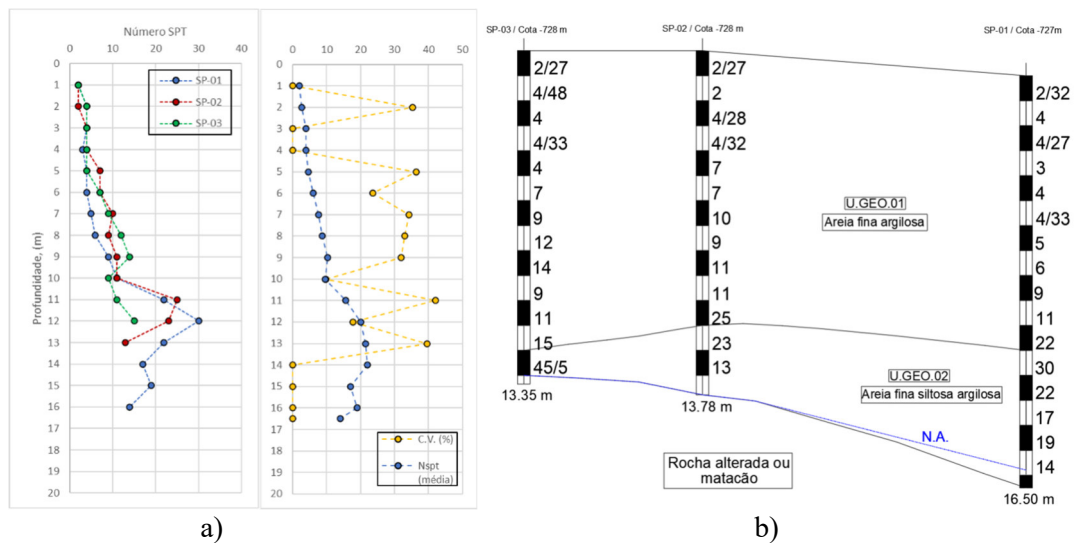
Figura 5. a) Resultados dos ensaios de campo ao longo do perfil do solo (SPT) de Itaipava/SP; b) Perfil geotécnico de Itaipava/SP.
