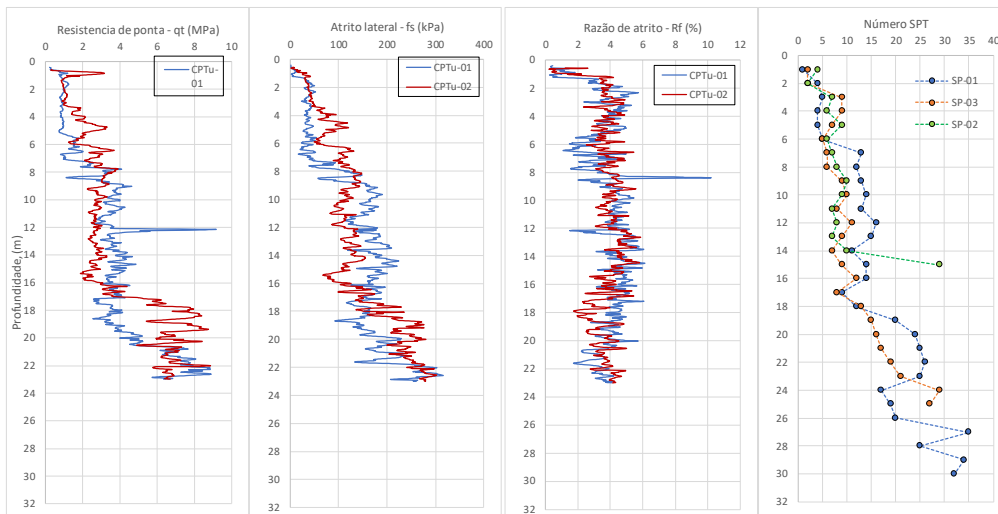
Figura 2. Resultados dos ensaios de campo ao longo do perfil do solo (SPT e CPTu) de Contagem/MG.
