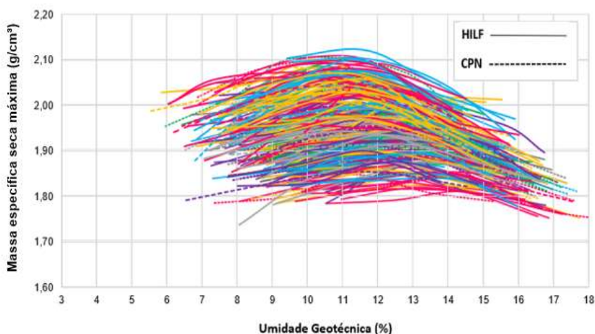
Figura 6 - Curva de compactação rejeito Brucutu
