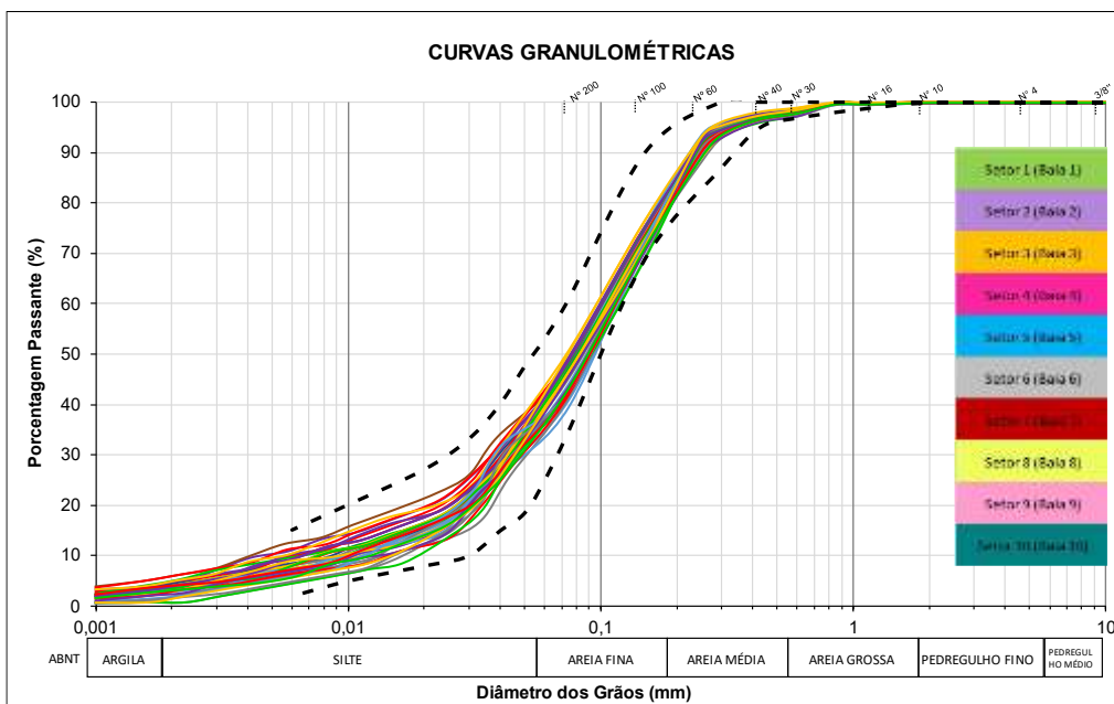
Figura 4 – Curvas granulométricas rejeito total Mina de Brucutu
