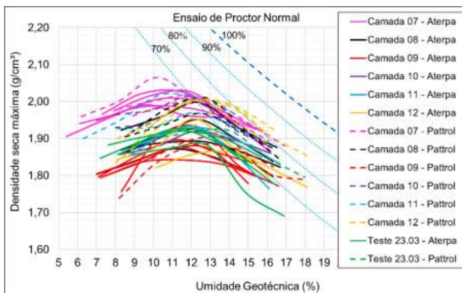
Figura 7 - Curva de compactação rejeito Itabira
