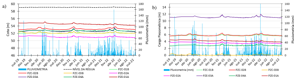
Figura 3. Seção A – Gráficos de a) Cota Piezométrica e b) Carga Piezométrica
