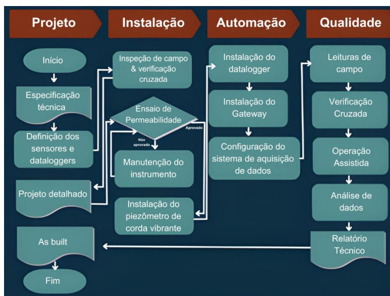
Figura 1. Processo esquemático da garantia da qualidade da instalação automatizada de piezômetros.
