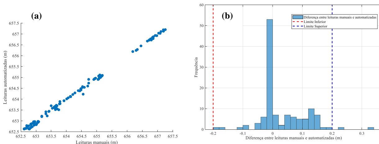
Figura 5. Relação entre a leitura manual e automatizada considerando todos os instrumentos analisados. (a) Gráfico de dispersão das leituras dos piezômetros manuais versus automatizados. (b) Histograma da diferença entre valores de leitura manual e automatizada.
