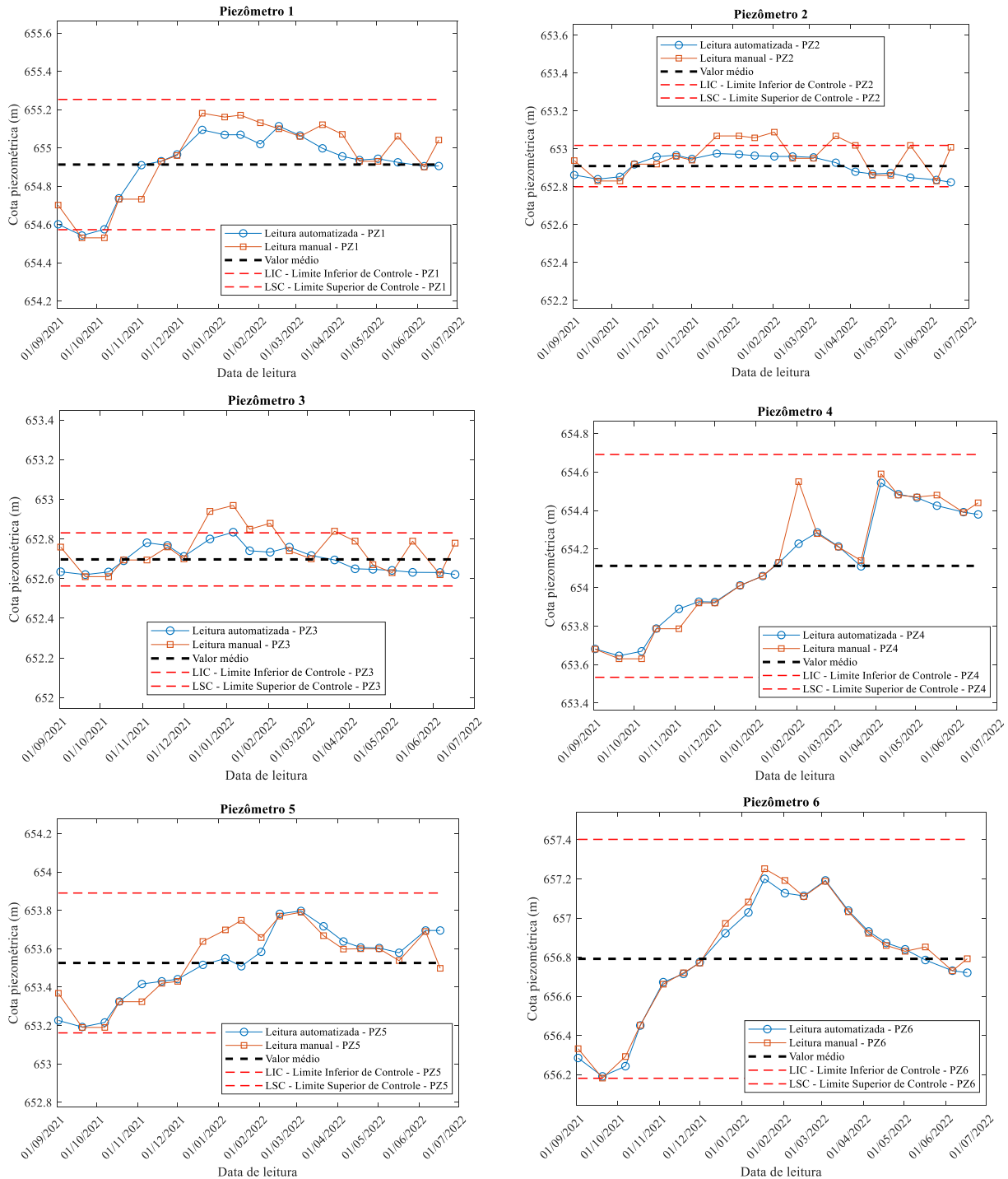
Figura 6. Comparação entre leituras manuais e automatizadas.
