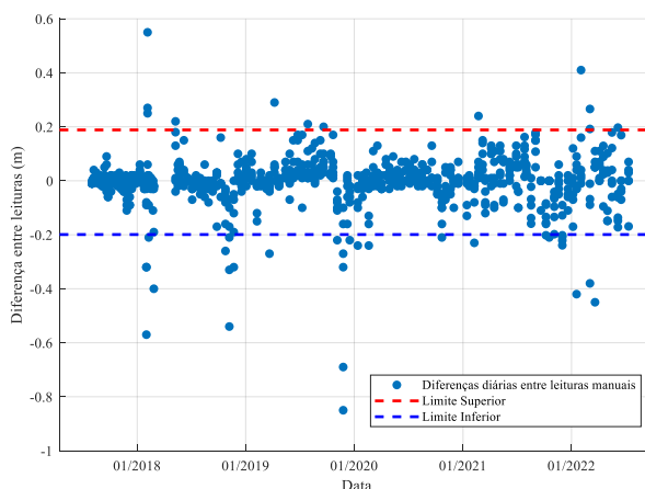
Figura 4. Série histórica de diferença entre leituras manuais.
