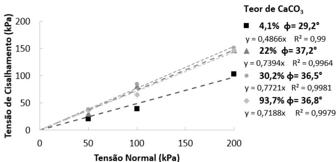
Figura 6 – Envoltória de ruptura e ângulos de atrito ( \phi ).
