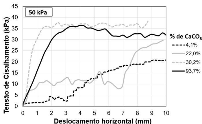
Figura 3 – Curvas de tensão de cisalhamento x deslocamento horizontal para tensão normal de 50 kPa.
