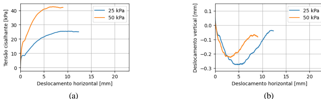
Figura 6. Ensaio de cisalhamento direto em amostra fofo sob tensões variadas para solo arenoso com adição de 10% de finos.
