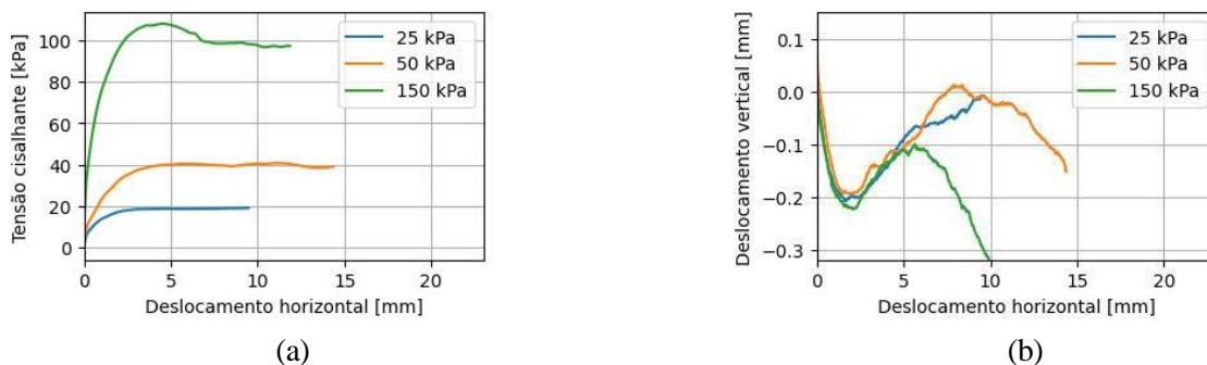
Figura 5. Ensaio de cisalhamento direto em amostra fofo sob tensões variadas para solo puramente arenoso.
