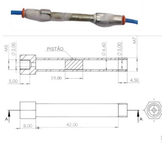
Figura 4. Areia colada com epóxi na parte central do cilindro do air hammer, teste de vedação e esquema com suas dimensões (mm)
