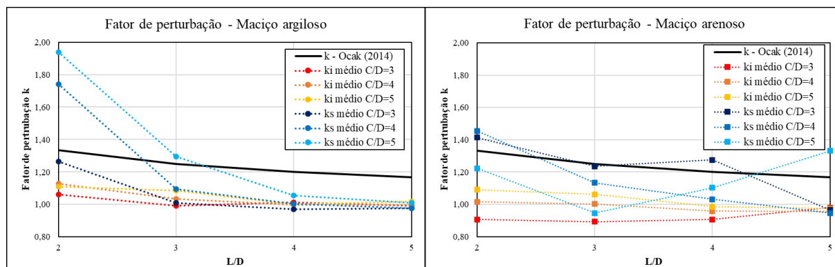
Figura 5. Comparação do fator de perturbação de Ocak (2014) para k_s e k_i
