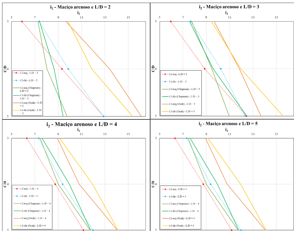
Figura 4. Valores de i_2 para o maciço arenoso
