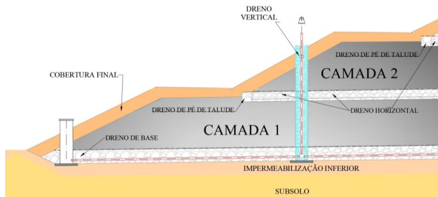
Figura 1. Esquema típico da rede de drenagem interna de lixiviado e biogás de aterros sanitários.
