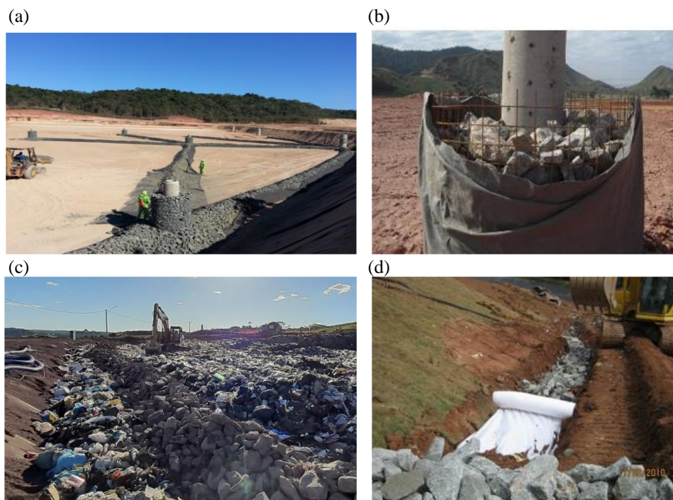
Figura 2. Imagens típicas de alguns tipos de drenagem interna de aterros sanitários: (a) Drenagem de base (no formato de espinha de peixe); (b) Drenagem vertical; (c) Drenagem horizontal (cortesia: Celso da Silva/CRVR); (d) Drenagem de pé de talude.
