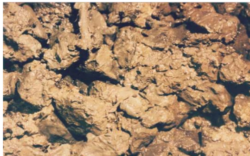
Figura 3. Camada drenante de base de aterro sanitário que não usou sistemas filtrantes em rachão (Fleming & Rowe 2004).
