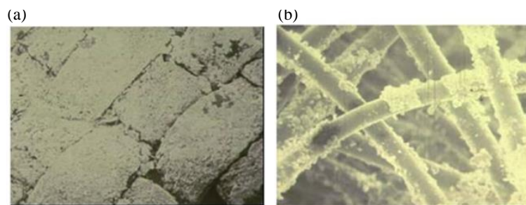
Figura 4 – Deposição biológica em geotêxteis aplicados em camadas drenantes de aterros sanitários botidas via microscopia: (a) geotêxtil tecido; (b) geotêxtil não tecido (Koerner e Koerner, 2015).
