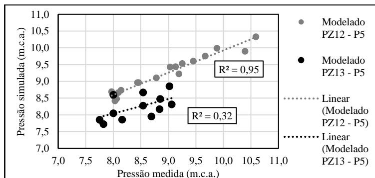
Figura 7. Correlação entre cotas piezométricas medidas e simuladas.
