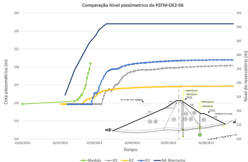
Figura 5- Comparação das cotas piezométricas medidas e das retroanálises realizadas do PZFM-DE2-06 com posição do ponto de medição em verde (seção B).
