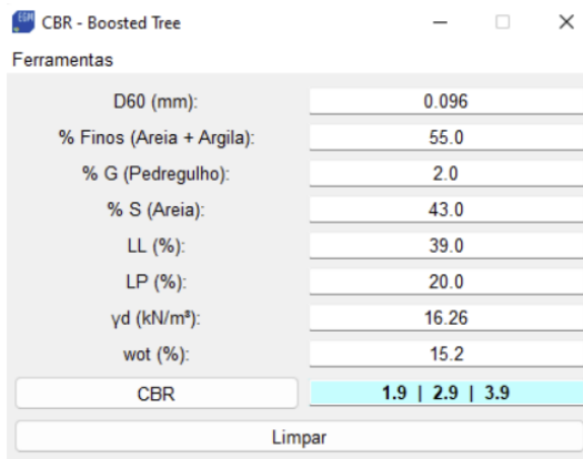
Figura 4. Programa em uso para obtenção do CBR.
