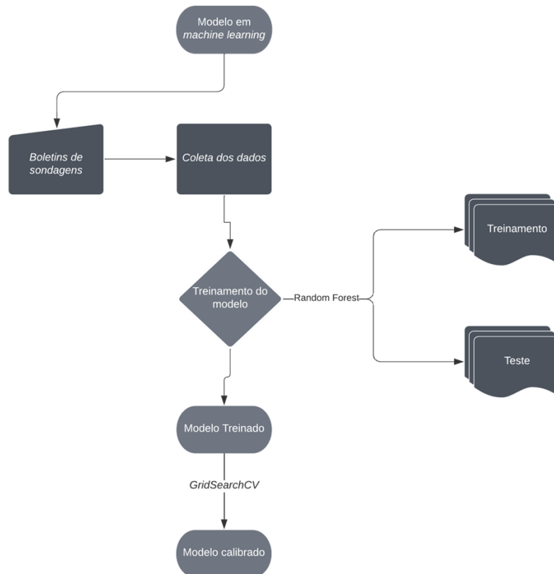
Figura 1. Fluxograma dos passos do trabalho
