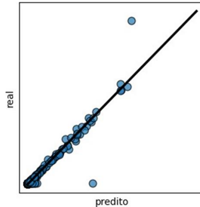
Figura 5. Correlação obtida para a sapata com B = 3,00 m
