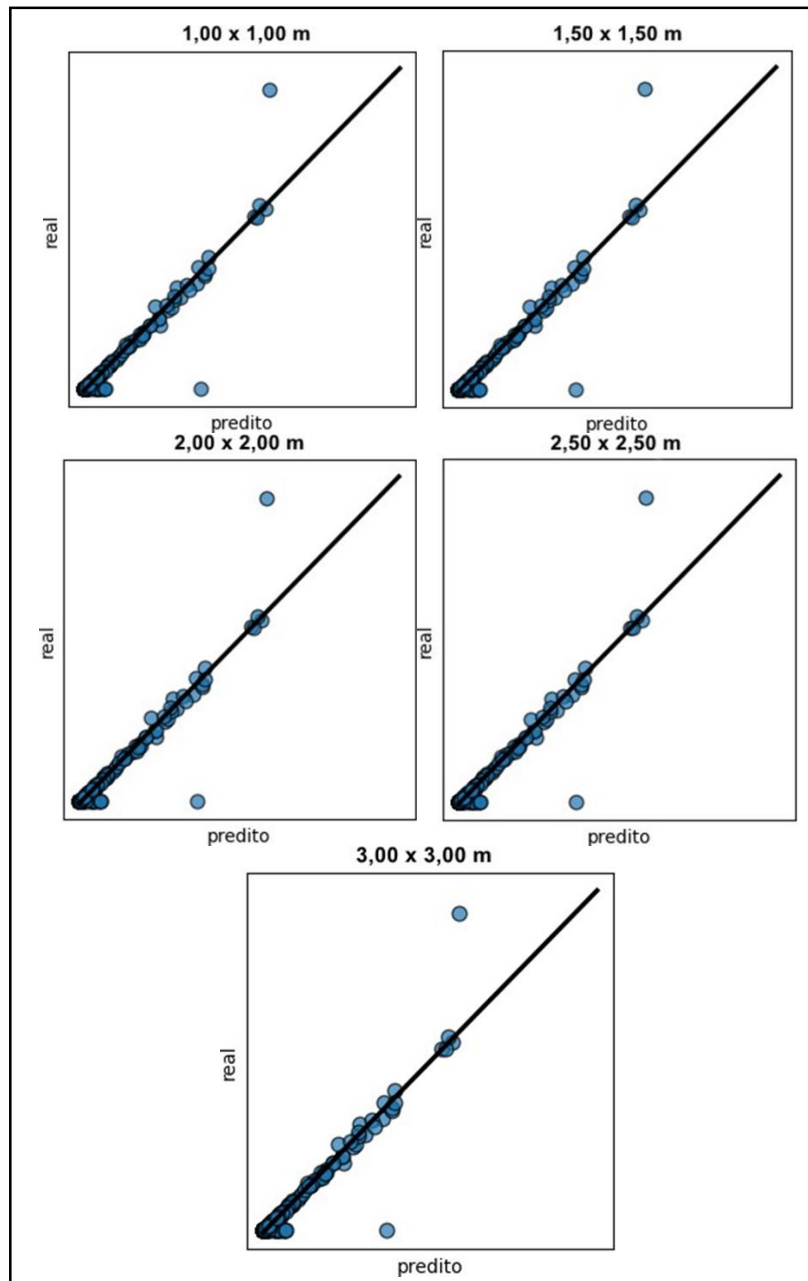
Figura 6. Valor predito vs. valor real do modelo obtido após a função GridSearchCV
