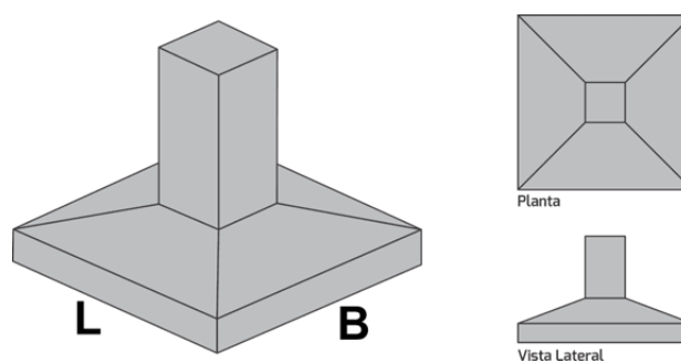
Figura 2. Esquema da sapata utilizada no modelo
