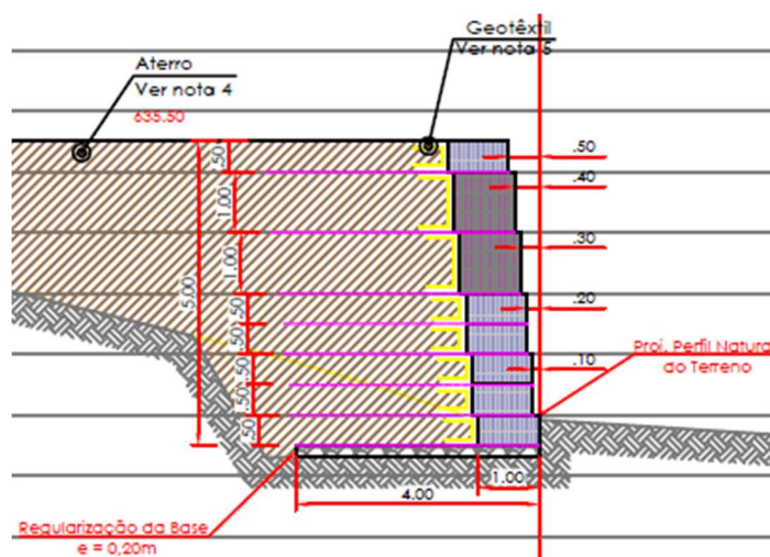
Figura 8. Seção tipo do Muro 2 com 5 m de altura Fonte: Projeto executivo da obra
