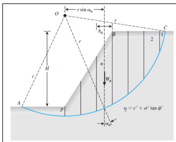
Figura 5 - Análise de um Talude Homogêneo pelo MEL
