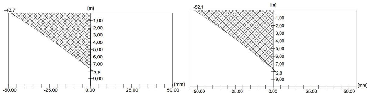
Figura 4 – Deslocamentos horizontais na cortina de estacas justapostas (à esquerda) e na cortina de estacas espaçadas (à direita) (GEO5, 2024).
