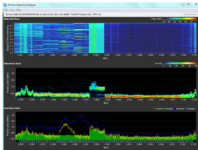
Figura 23 – Tela do Analisador de Espectro Teixeira de Freitas.
