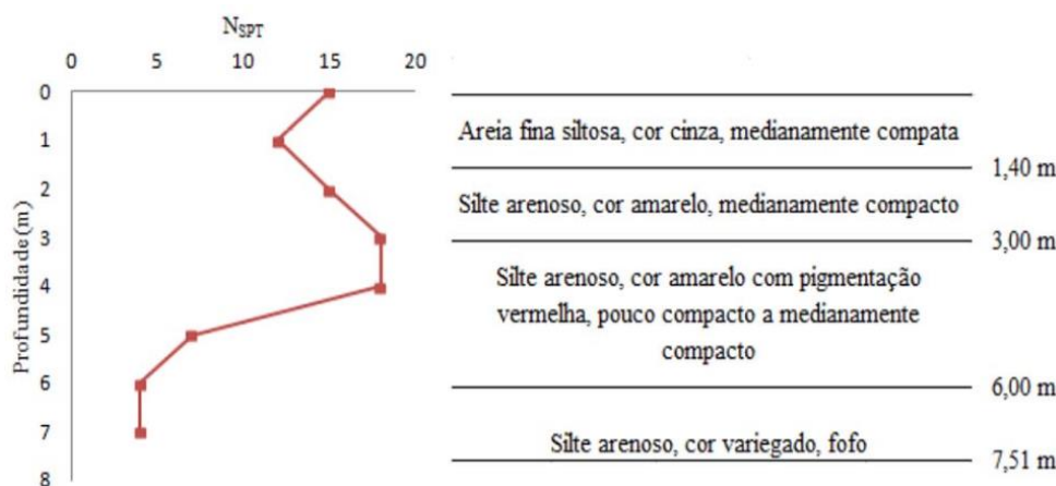
Figura 2. Resultado da sondagem à percussão realizada (Fonte: MOURA et. al., 2018).
