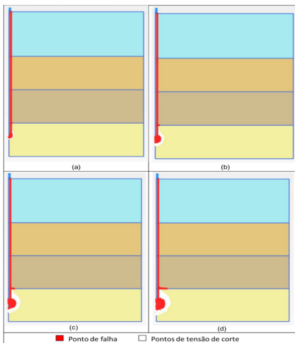
Figura 5 – Pontos plásticos nos estágios de carregamento a) 5, b) 9, c) 14 e d) 18 -PCE-02
