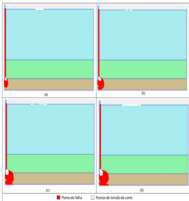
Figura 7 – Pontos plásticos nos estágios de carregamento a) 5, b) 9, c) 14 e d) 18 -PCE-01
