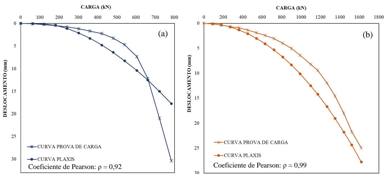
Figura 3 – Comparação entre curvas carga vs recalque obtidas por modelagem numérica com curva obtida por meio de prova de carga estática - (a) PCE-01 (b) PCE-02
