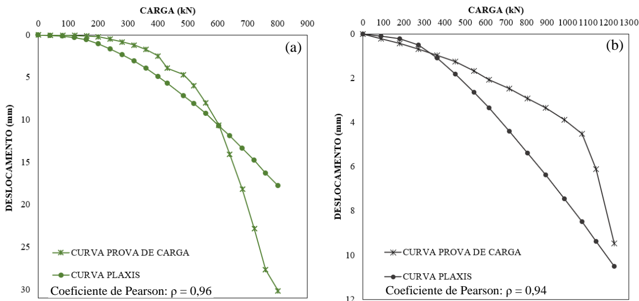
Figura 6 – Comparação entre curvas carga vs recalque obtidas por modelagem numérica com curva obtida por meio de prova de carga estática - (a) PCE-03 (b) PCE-04
