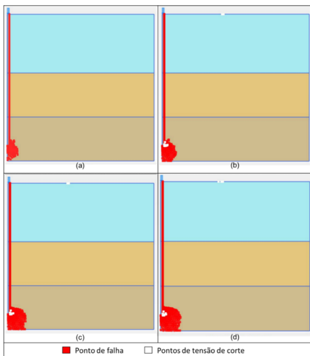
Figura 4 – Pontos plásticos nos estágios de carregamento a) 5, b) 9, c) 14 e d) 18 -PCE-01
