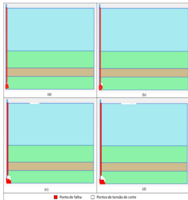
Figura 8 – Pontos plásticos nos estágios de carregamento a) 5, b) 9, c) 14 e d) 18 -PCE-02
