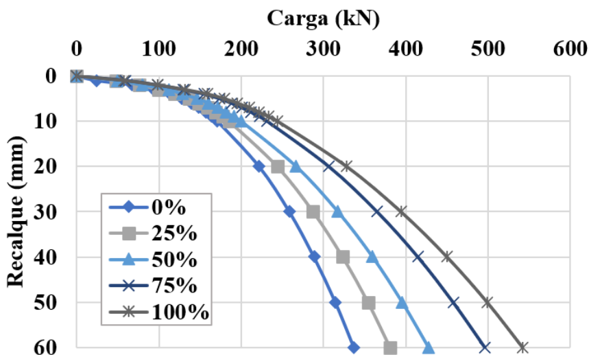
Figura 4. Comportamento carga versus recalque das fundações estacadas em relação a diferentes percentuais do cobrimento.
