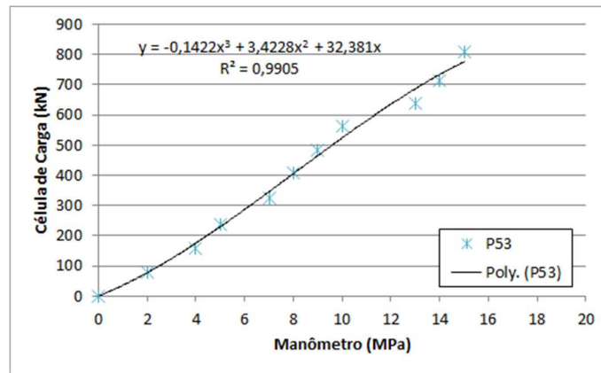
Figura 8. Regressão polinomial da prova de carga P53
