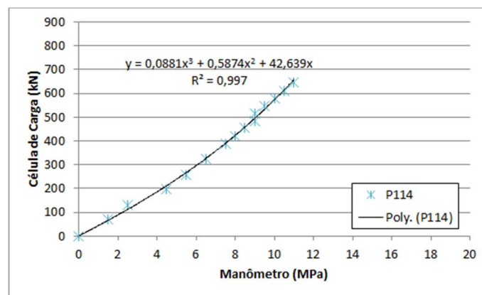
Figura 9. Regressão polinomial da prova de carga P114
