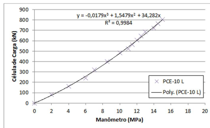
Figura 6. Regressão polinomial da prova de carga PCE-10L
