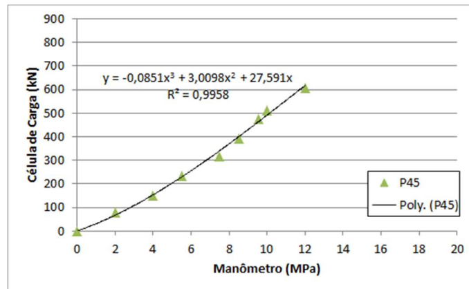
Figura 5. Regressão polinomial da prova de carga P45
