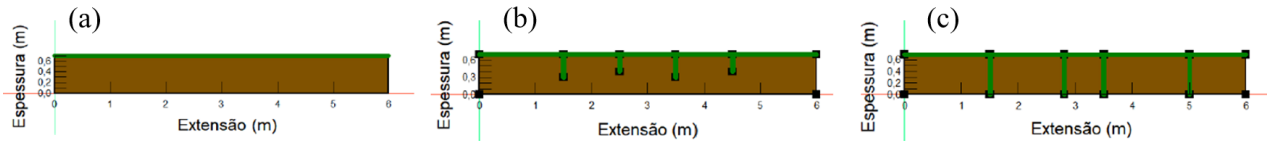
Figura 1. Camadas de cobertura modelo (a) sem fissura (b) com fissura até metade da profundidade (c) fissura até o limiar da camada.
