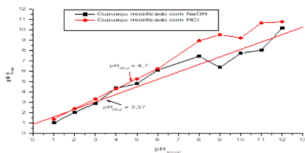
Figura 1: Ponto de Carga Zero (PCZ) das biomassas em estudo
