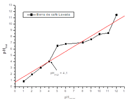
Figura 1: Ponto de Carga Zero (PCZ) Borra de Café Lavada
